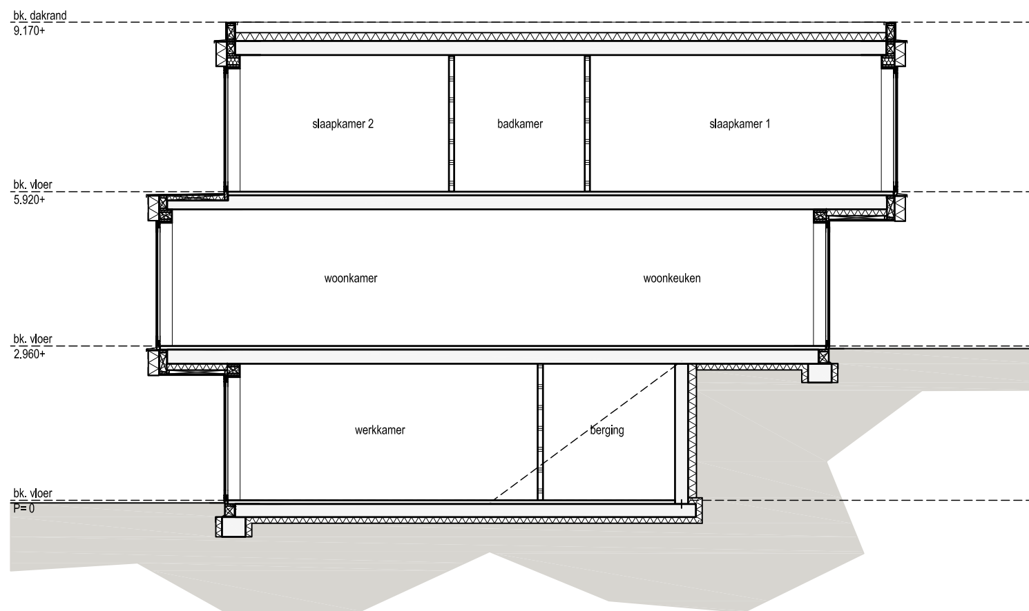
DOORSNEDE
