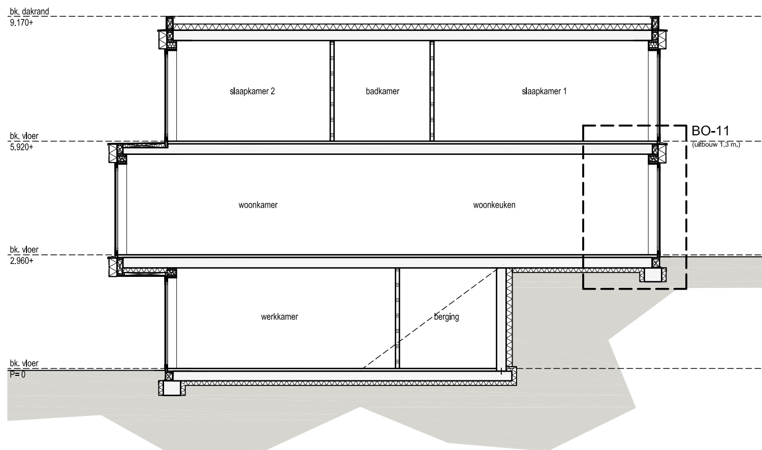
DOORSNEDE
